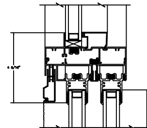
2 TRANSOM PB200
