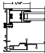
4 LOCK JAMB PB200
