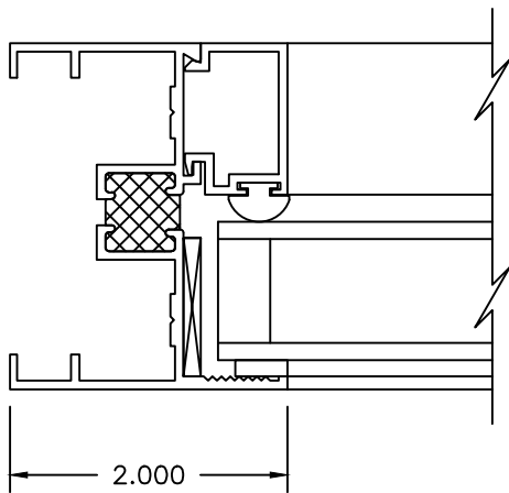
④ LEFT JAMB FIXED
