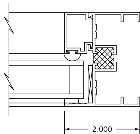
④ OPP RIGHT JAMB FIXED
