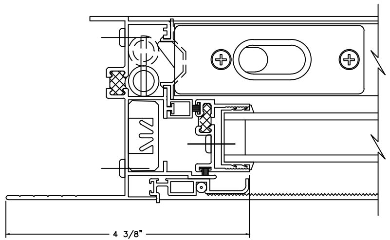
④ FLANGED JAMB DH
