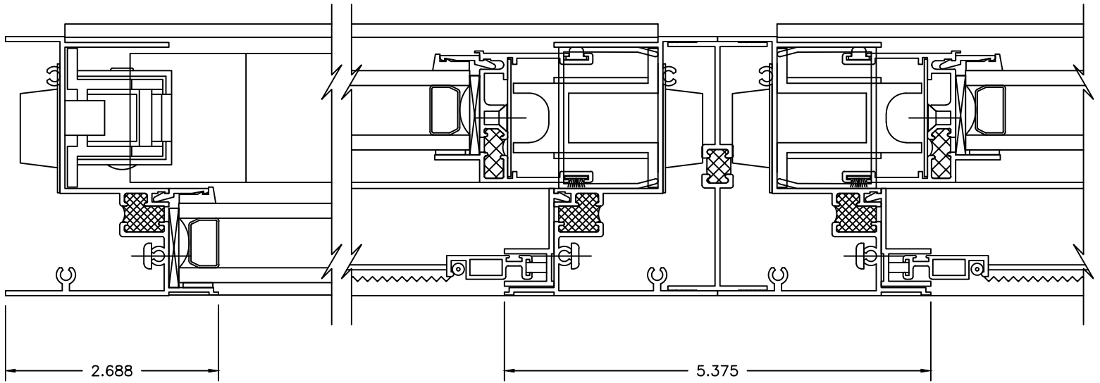
④ LEFT JAMB RIGHT JAMB(OPPOSITE)
