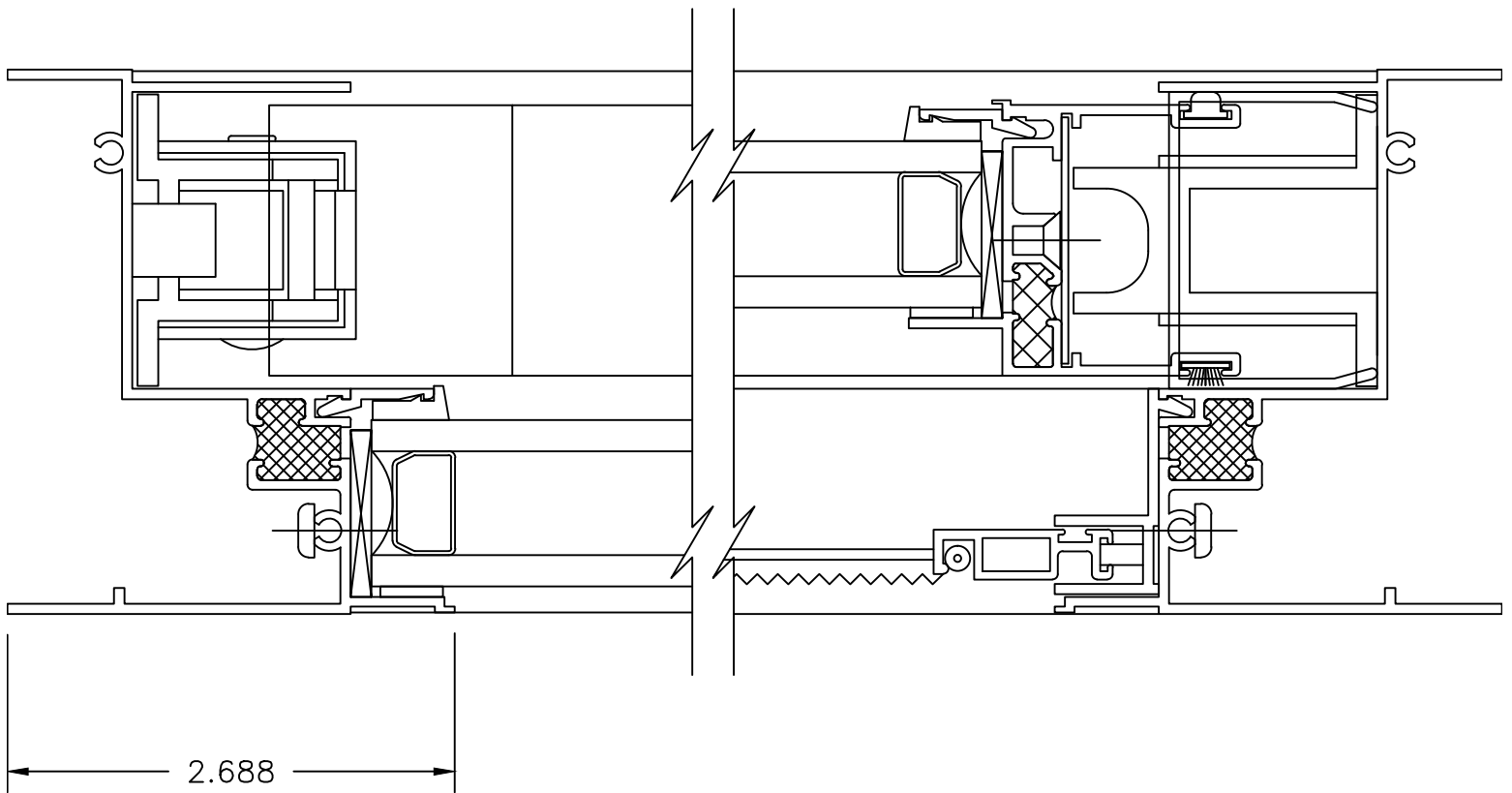
④ LEFT JAMB
