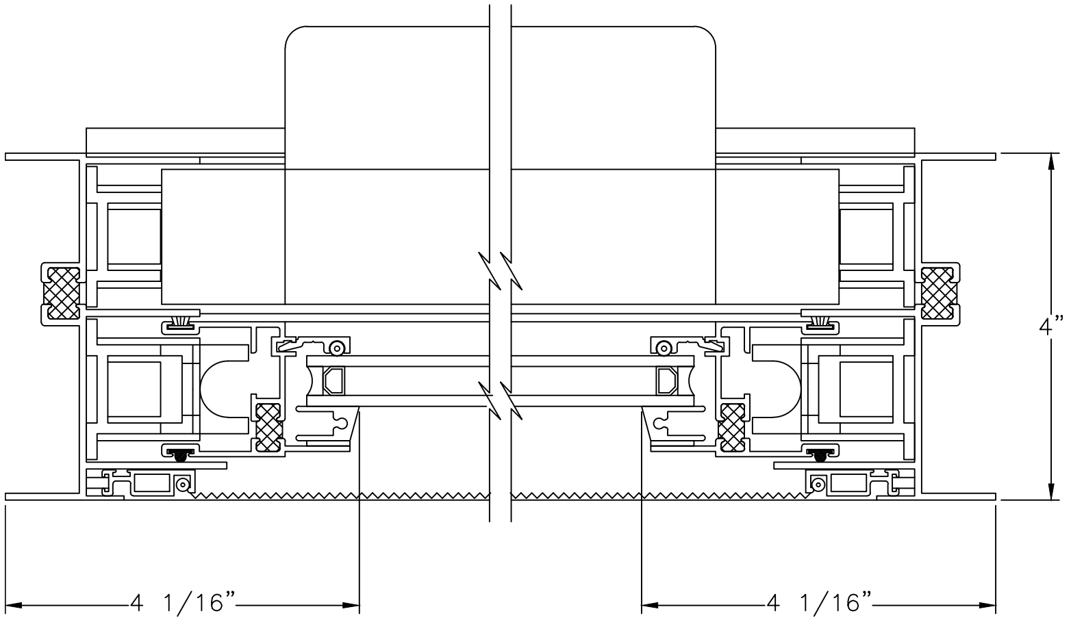
④ LEFT JAMB P4300 DH
