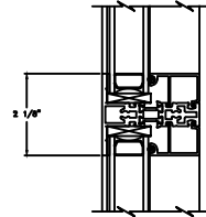
13 HORIZ TRUE MUNTIN P6100
