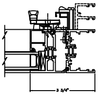
8 CASEMENT RIGHT JAMB P6100
