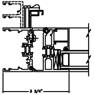
7 CASEMENT LEFT JAMB P6100
