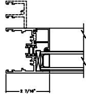
3 FIXED LEFT JAMB P6100
