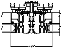
15 CASEMENT VERT INT MULLION P6100
