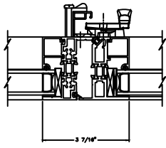
9 CASEMENT VERT INT MULLION P6100
