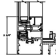
6 CASEMENT SILL P6100
