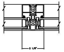
14 VERT TRUE MUNTIN P6100
