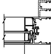
4 FIXED RIGHT JAMB P6100
