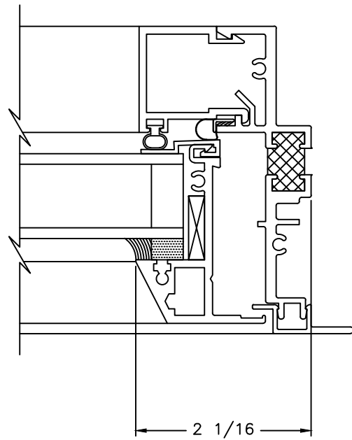
⑥ RIGHT JAMB P7500
