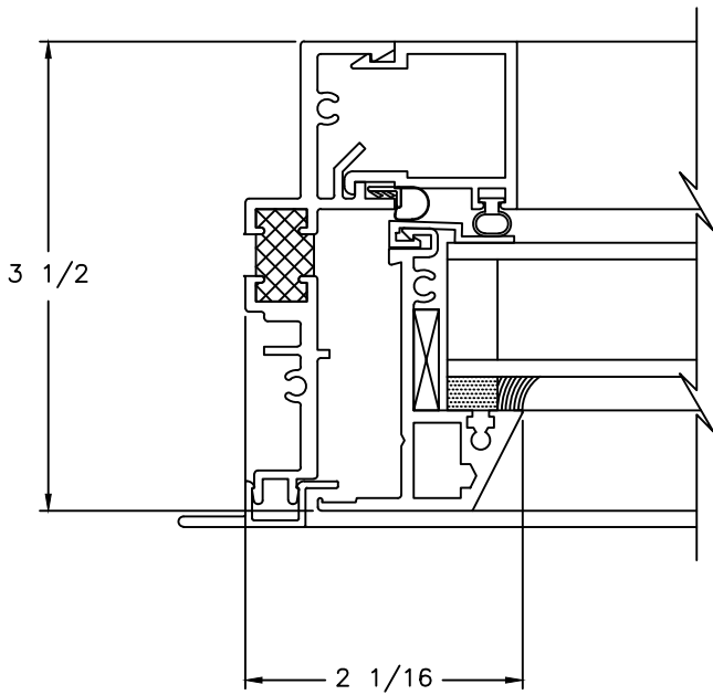
④ LEFT JAMB P7500
