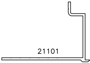
#2 JAMB PANNING 1 1/4" PROJ. X 2 1/2" LEG
