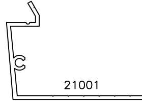
#2 HEAD & SILL PANNING 1 1/4" PROJ. X 2 1/2" LEG
